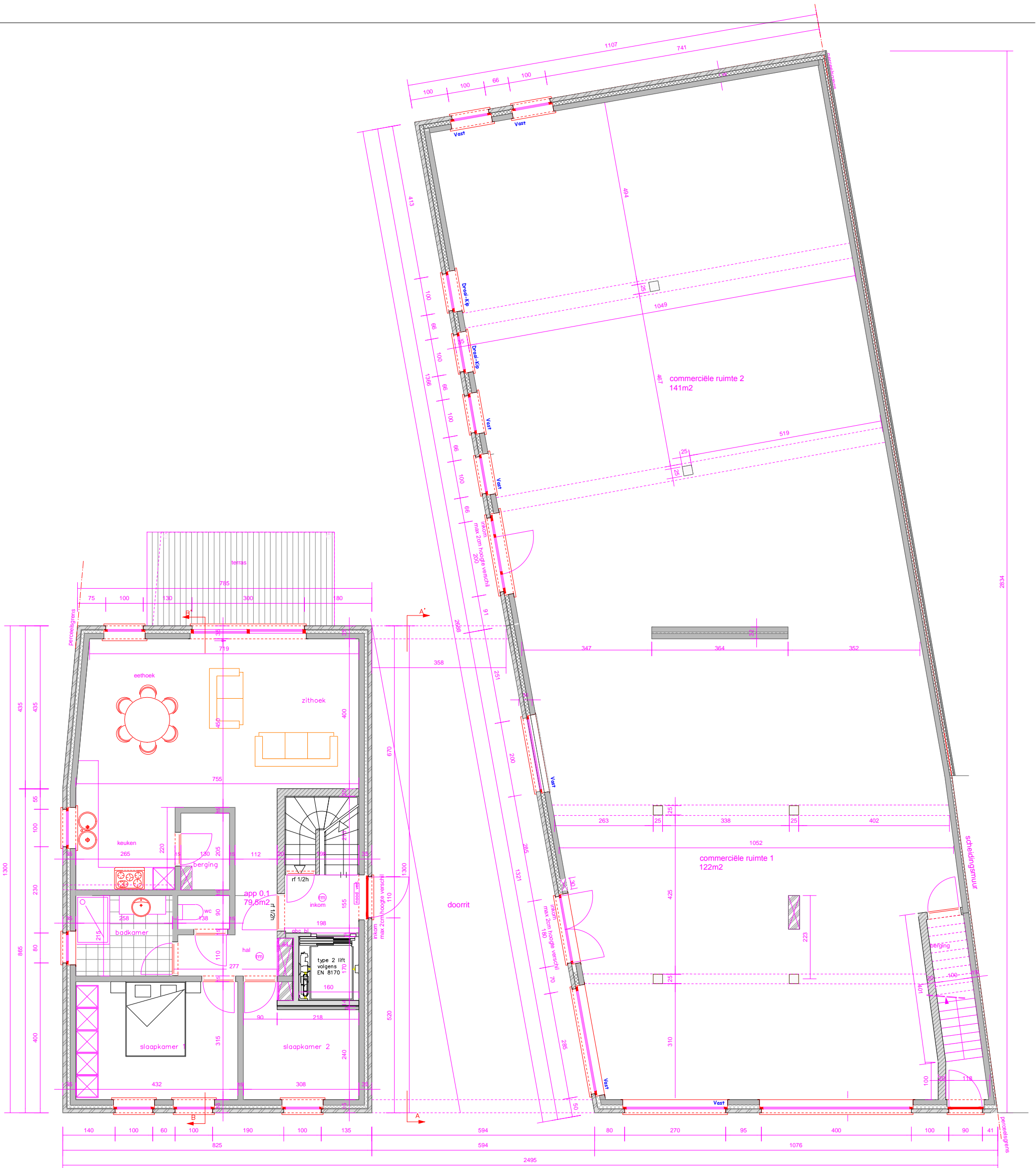
GRONDPLAN
